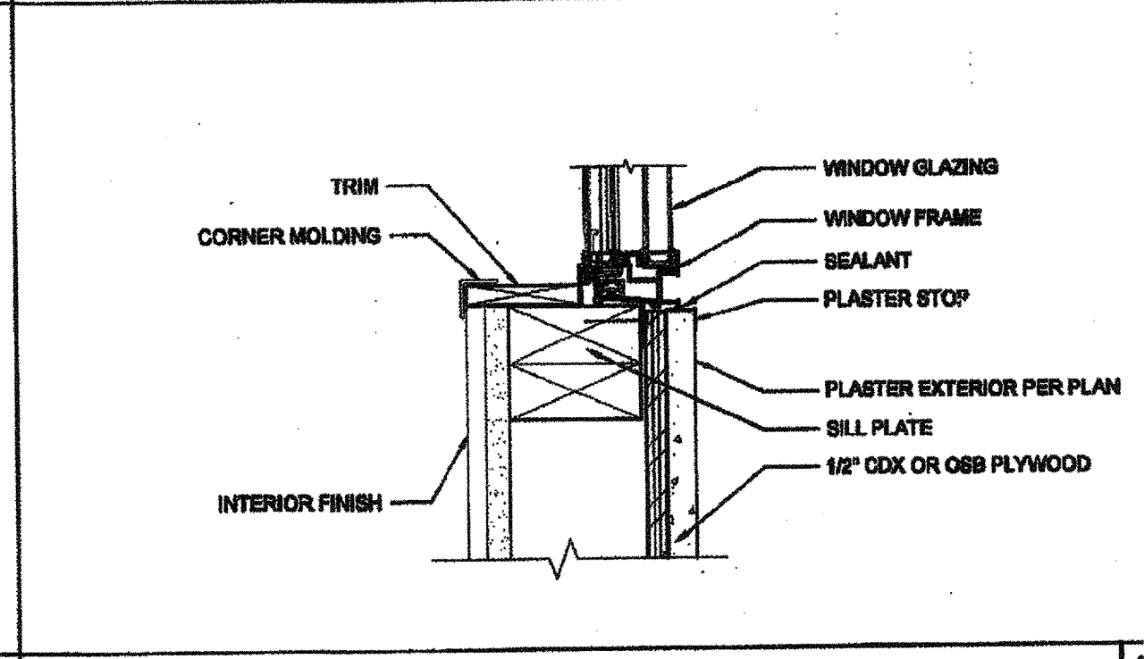
WINDOW SILL SCALE: 3/4"=1'-0" 13
