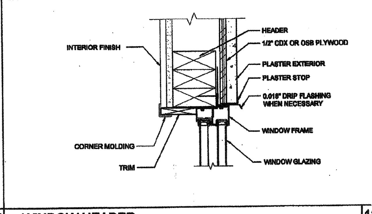
WINDOW HEADER SCALE: 3/4"=1'-0" 12
