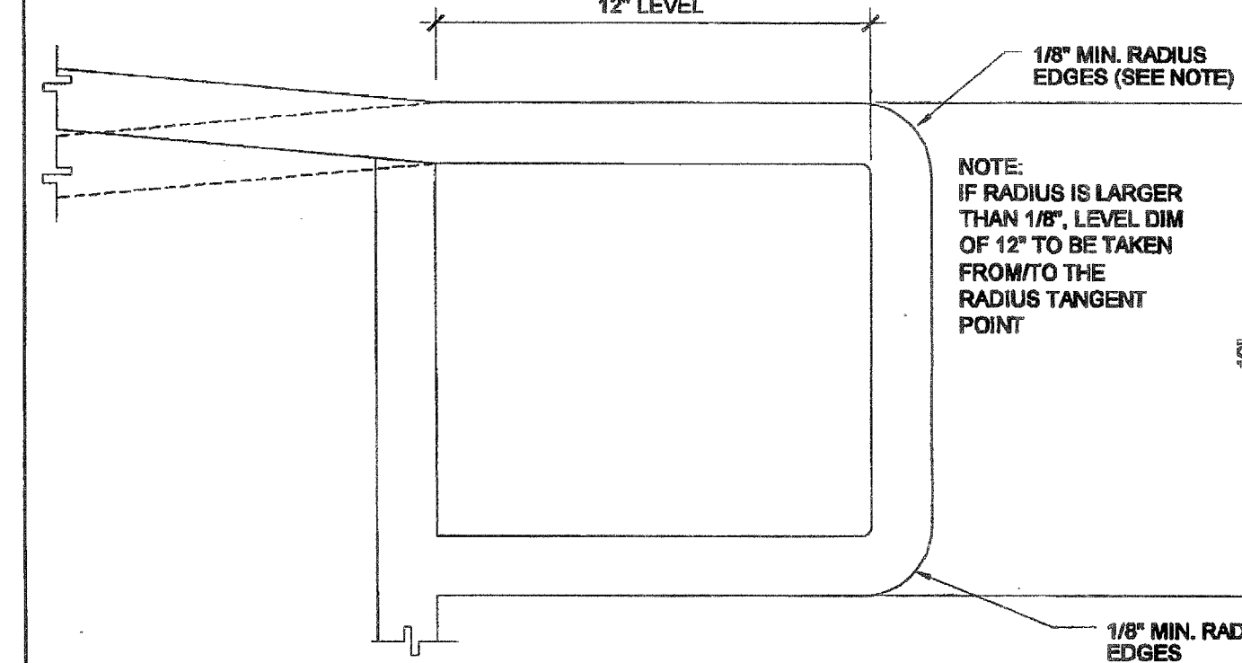
RAMP EXTENSION SCALE: 6" = 1'-0" 8
