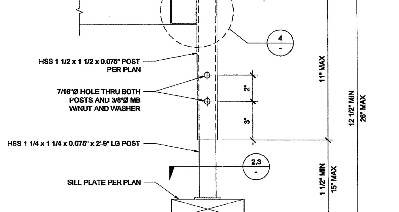
ADJUSTABLE LEG SCALE: 3" = 1'-0" 1
