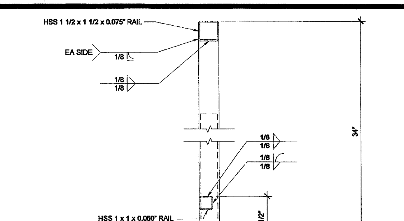
ADJUSTABLE LEG SCALE: 3" = 1'-0" 1
