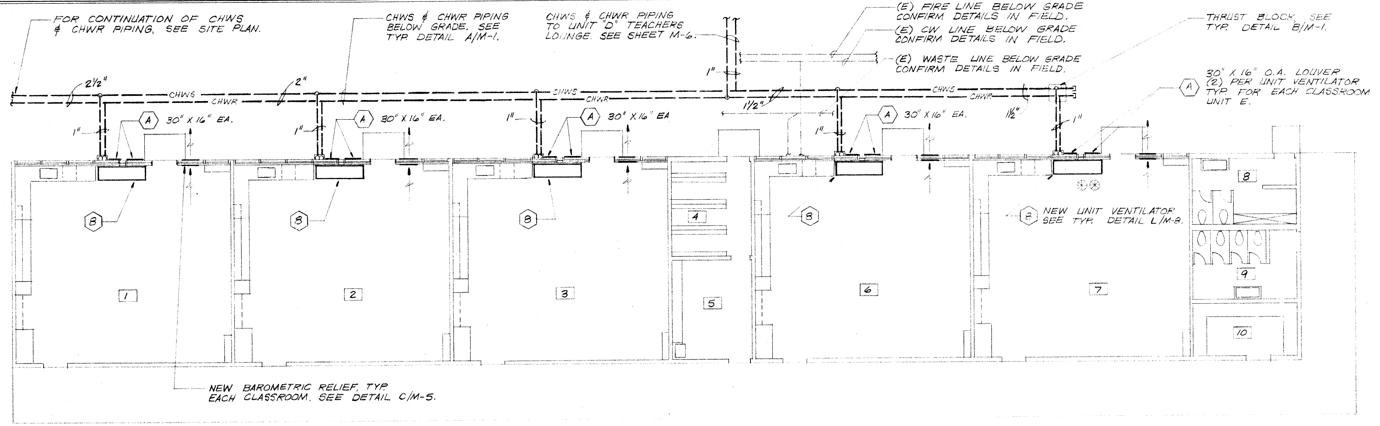
UNIT E AIR CONDITIONING PLAN SCALE: 1/8" = 1'-0"
