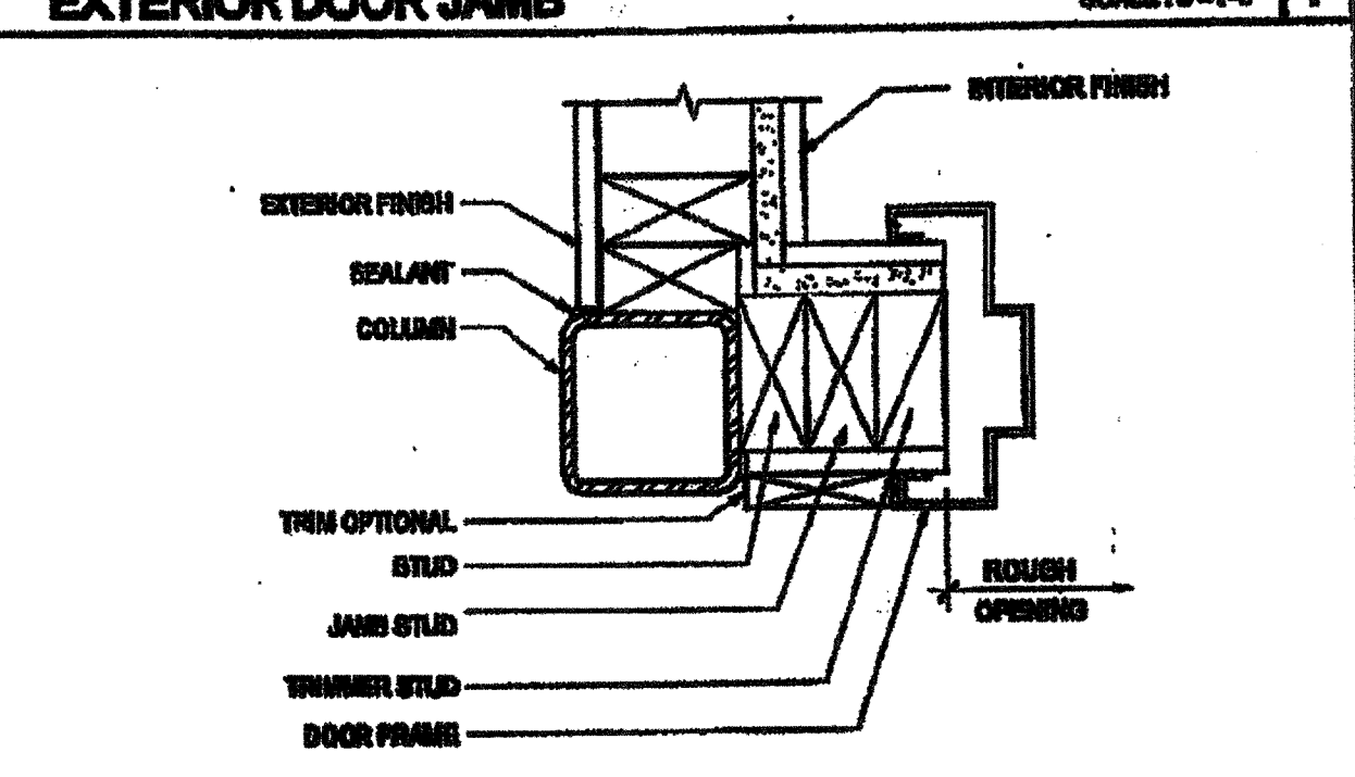
EXTERIOR DOOR JAMB SCALE: 1/2"=1'-0" 8
