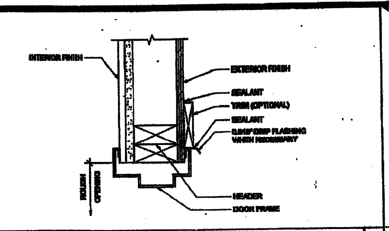
EXTERIOR DOOR HEADER SCALE: 1/2"=1'-0" 6
