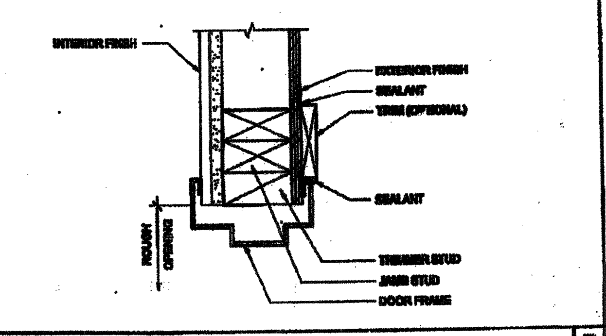
EXTERIOR DOOR JAMB SCALE: 1/2"=1'-0" 7
