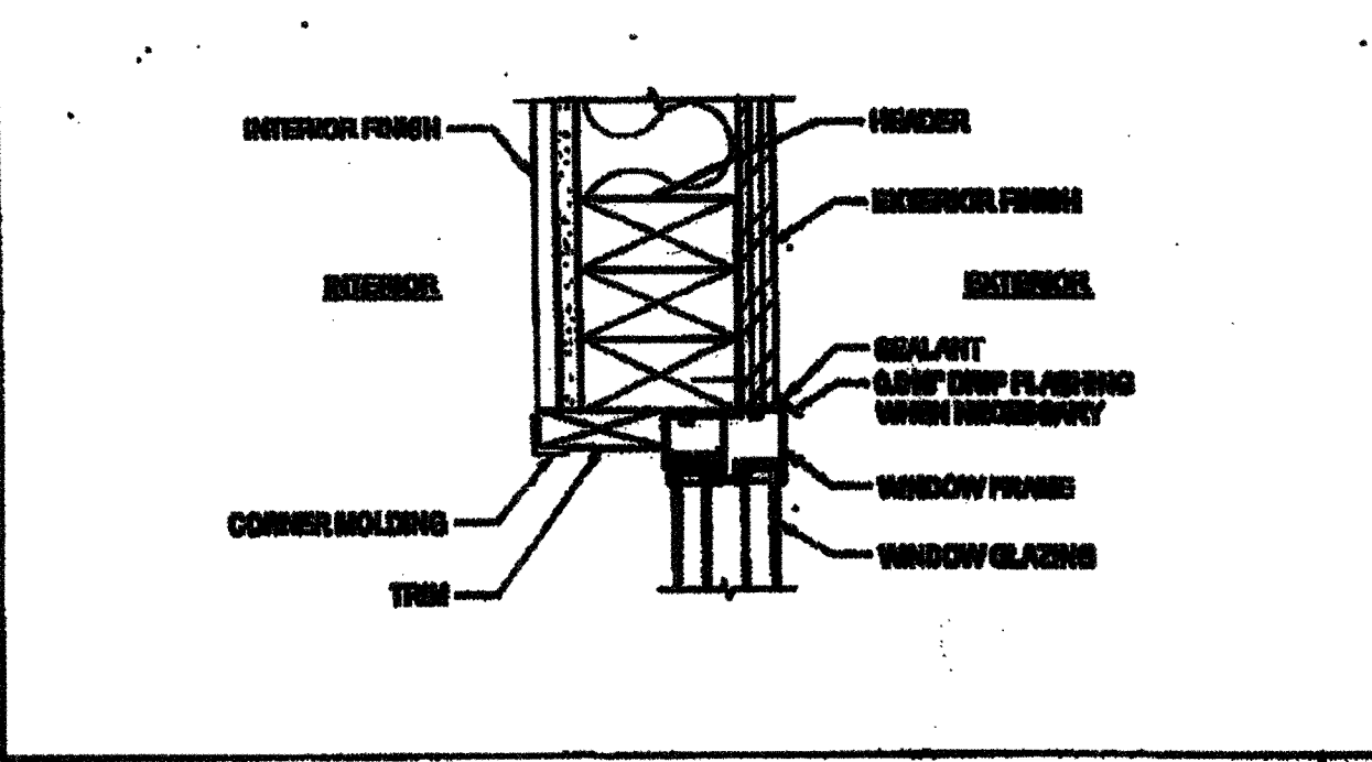
WINDOW HEADER SCALE: 1/2"=1'-0" 12
