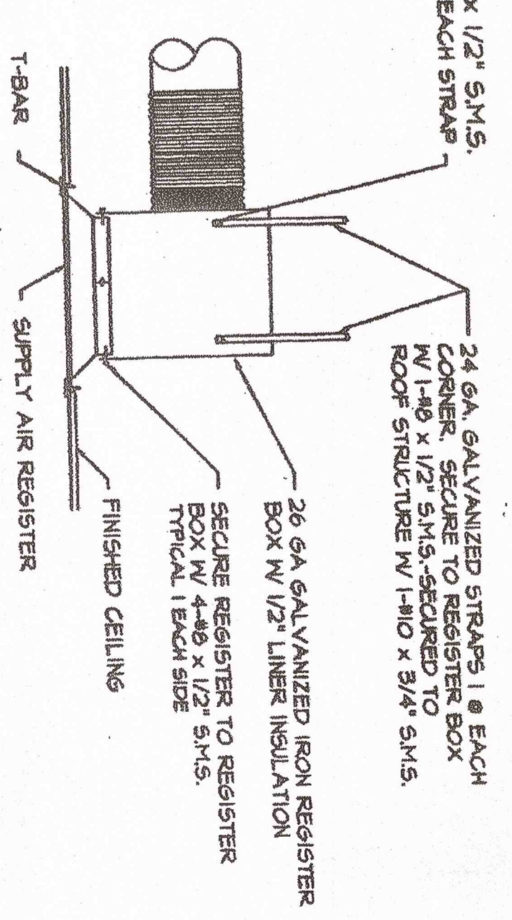
REGISTER BOX DETAIL N.T.S.
