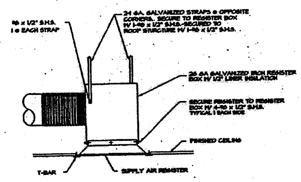
REGISTER BOX DETAIL N.T.S.
