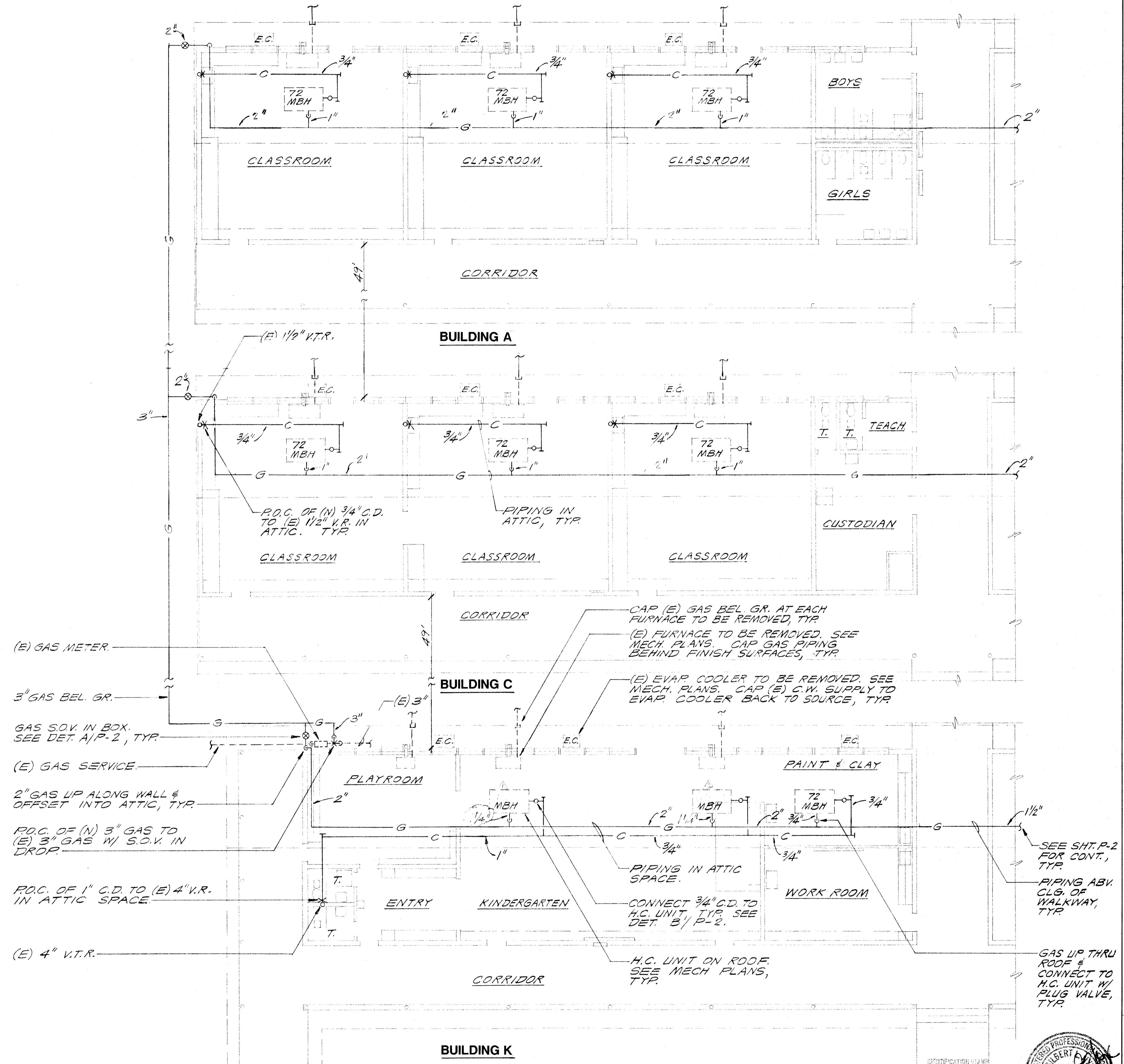
PLUMBING PLAN SCALE: 1/8" = 1'-0"
