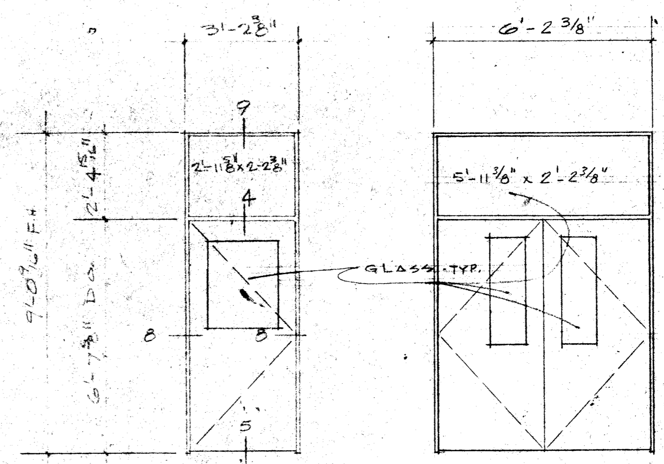
DOOR ASSEMBLY
