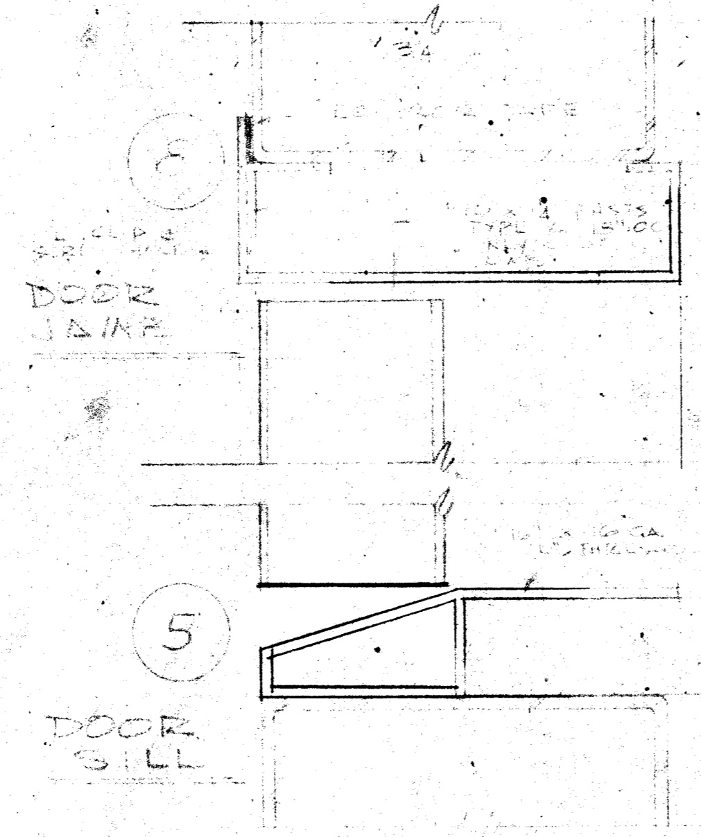
DOOR SECTIONS
