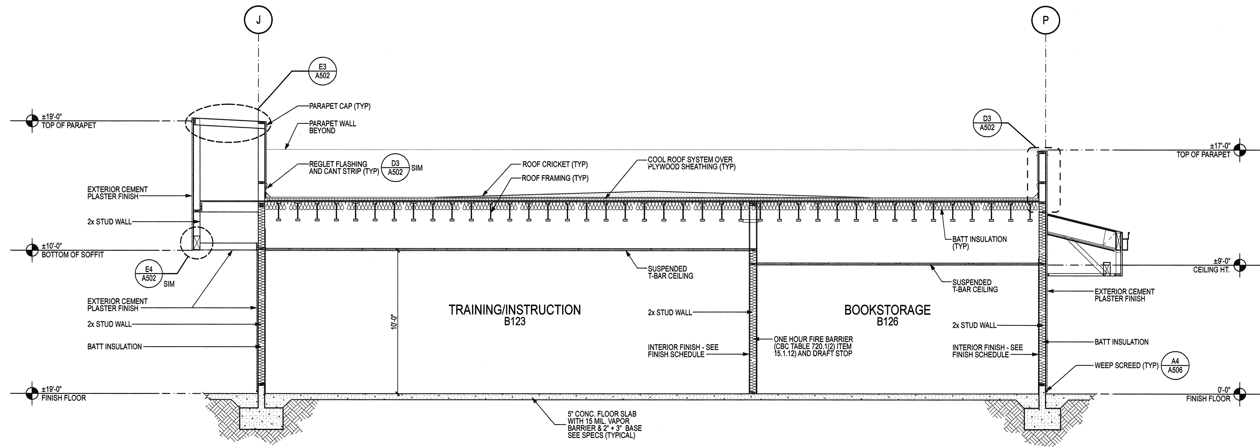
D1 BLDG B SECTION SCALE: 1/4" = 1'-0"
