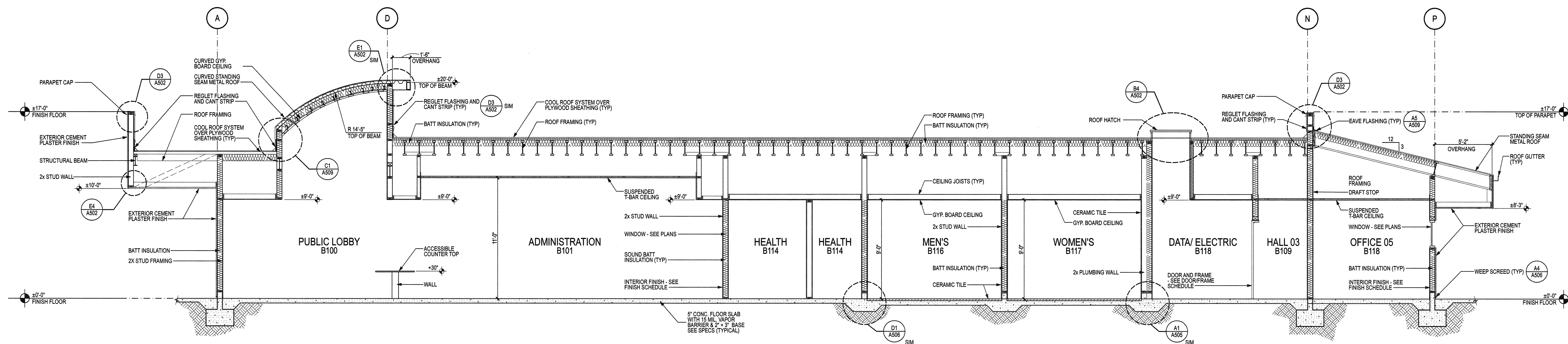
D1 BLDG B SECTION SCALE: 1/4" = 1'-0"
