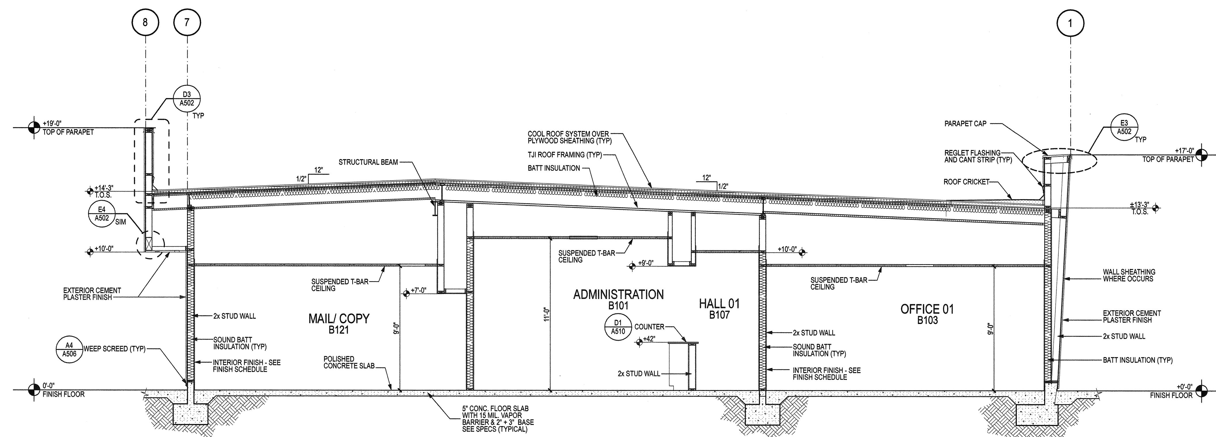
D1 BLDG B SECTION
