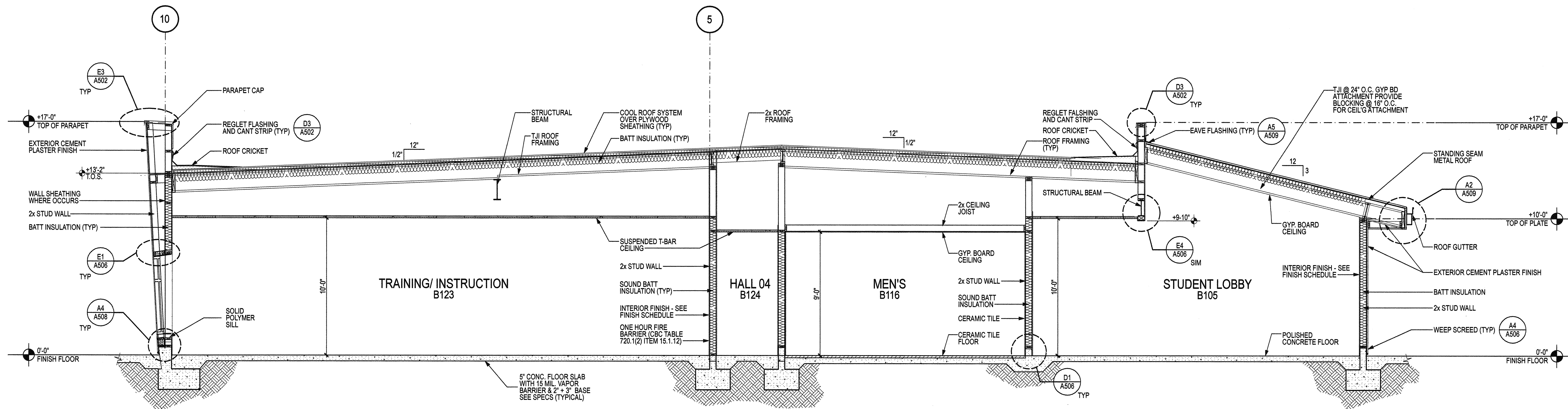
D1 BLDG B SECTION
